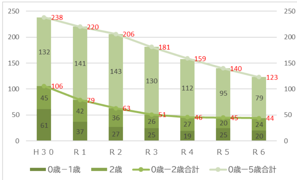
■ 0 - 2 歳、3 - 5 歳のこどもの人口 (各年 4 月 1 日現在) 単位：人
